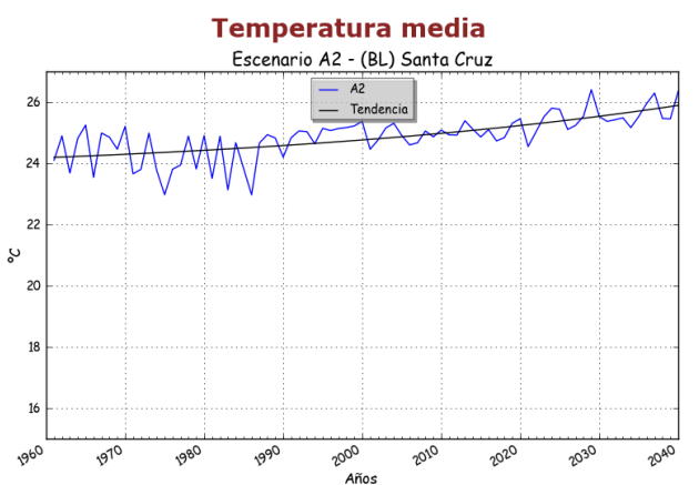
Figura 65: Tendencia de la temperatura media anual (1961-2040): Escenario A2, Bolivia
