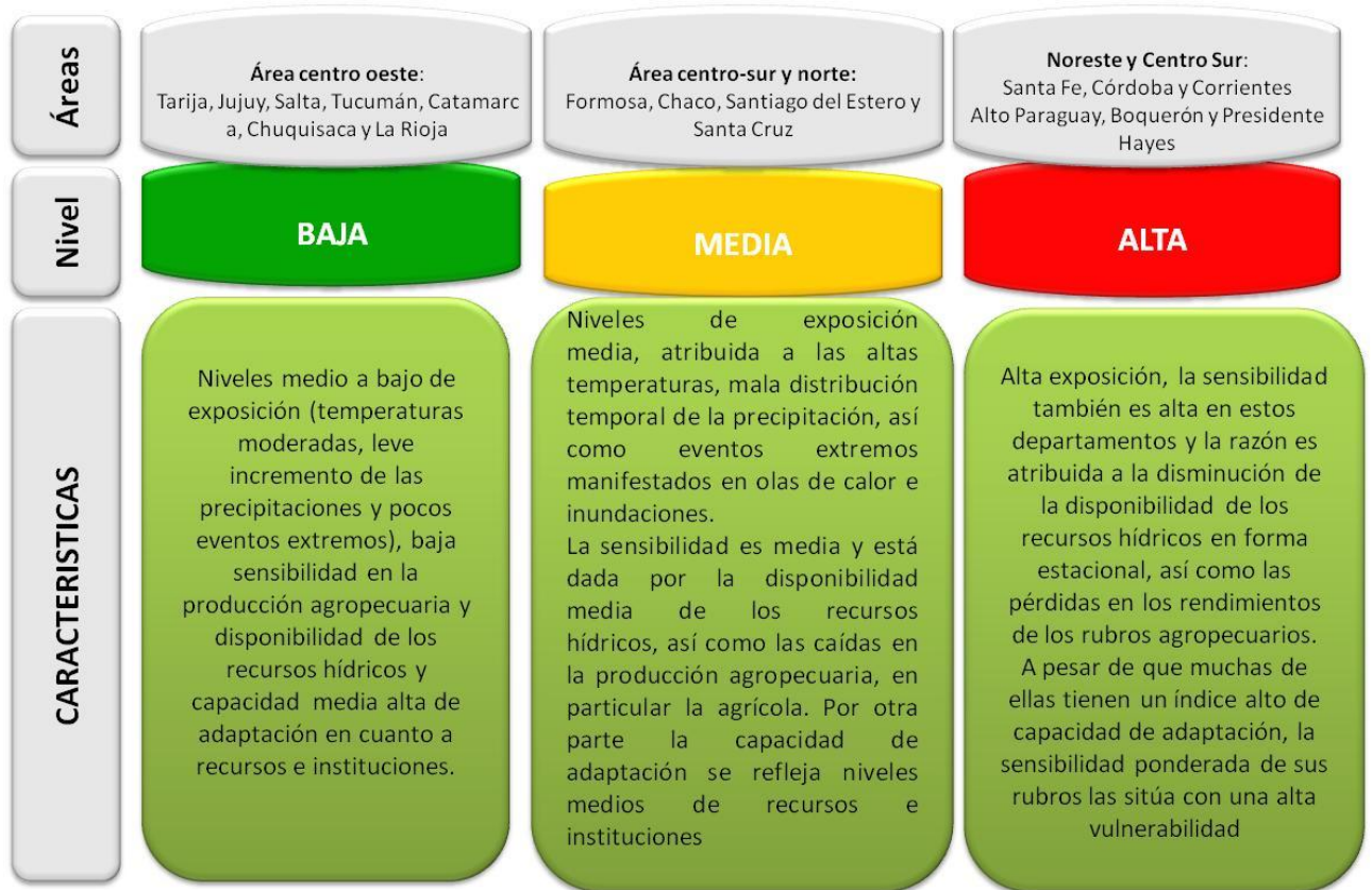
Figura 152: Resultados de la vulnerabilidad regional 2011-2040
