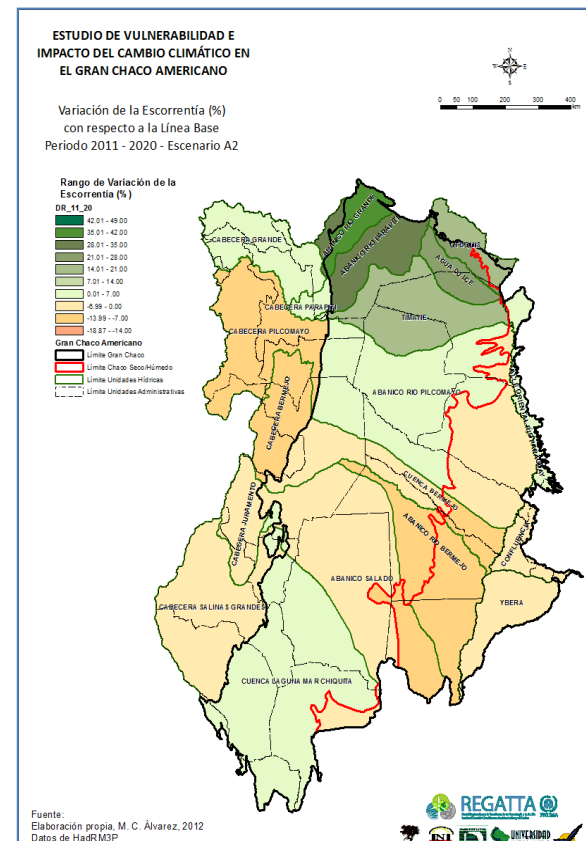
Figura 101: Variación de la Escorrentía 2011-2020 (%)
