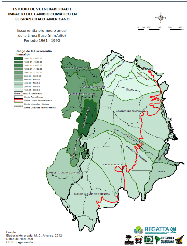
Figura 80: Escorrentía 1961- 1990. (mm)
