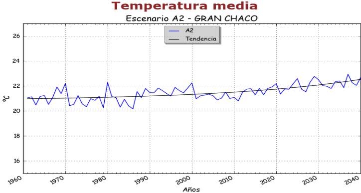
Figura 63: Tendencia de la de la temperatura media en el Gran Chaco para el escenario A2
